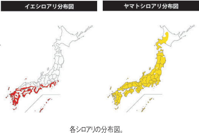
各シロアリの分布図。
